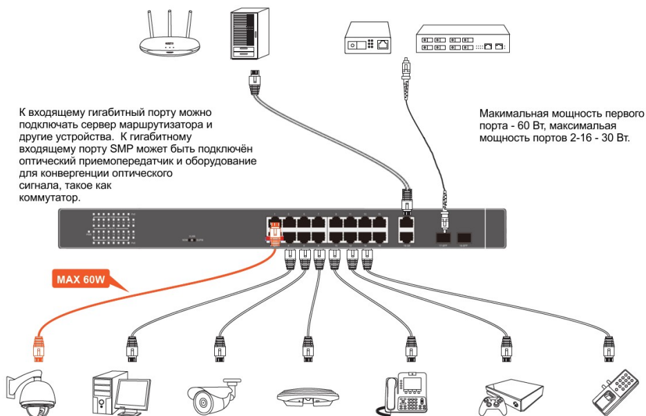
Рисунок 6 – Схема подключения устройств к коммутатору
